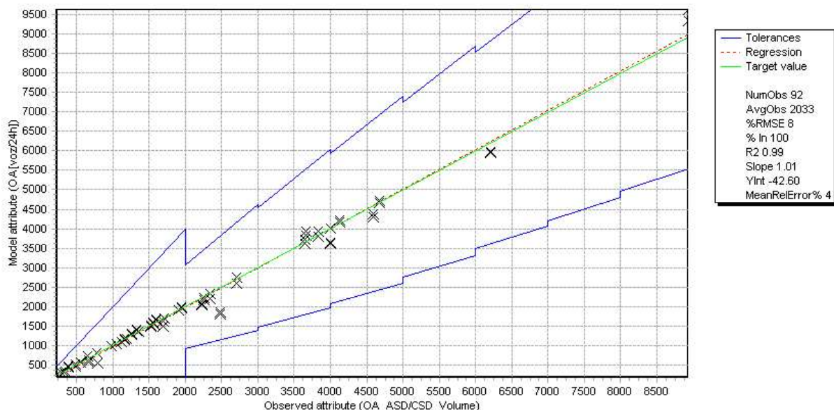
Obrázok 9 Kvalita kalibrácie zaťaženia siete osobnými automobilmi
